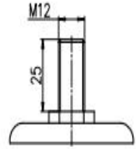
丝杆
