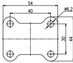
平板定向
