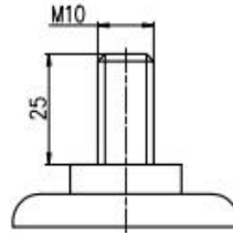
丝杆
